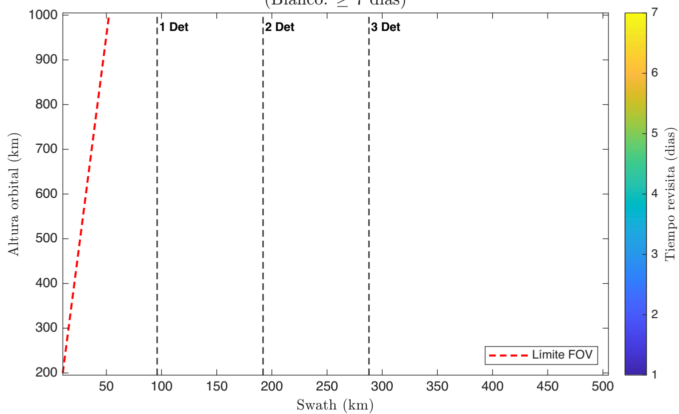
Tiempo Revisita - 3 Satellite(s); 1 Telescopio(s): Cassegrain; Detector 1 (Blanco: \geq 7 dias)
